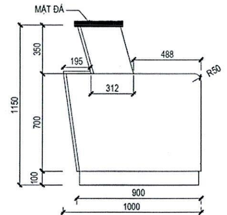
CHI TIẾT MẶT CẮT DỌC HÔNG
