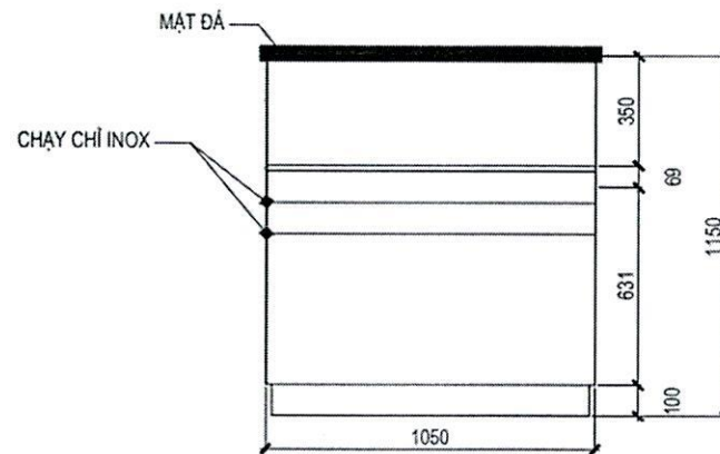
CHI TIẾT MẶT ĐỨNG TRƯỚC
