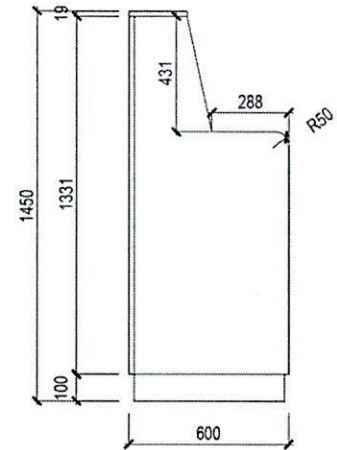
CHI TIẾT MẶT CẮT DỌC HÔNG
