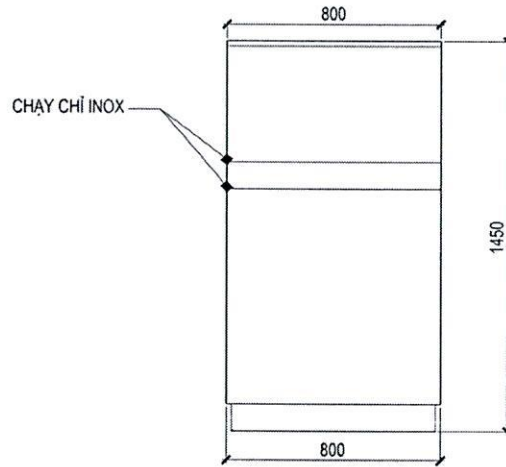
CHI TIẾT MẶT ĐỨNG TRƯỚC
