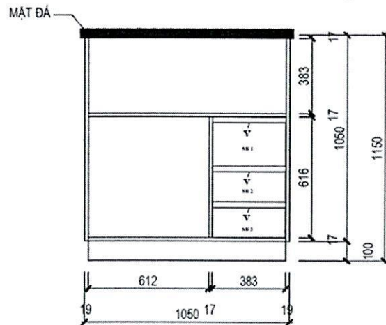
CHI TIẾT MẶT ĐỨNG SAU
