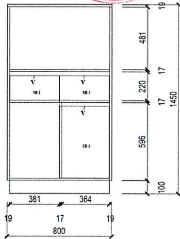
CHI TIẾT MẶT ĐỨNG SAU
