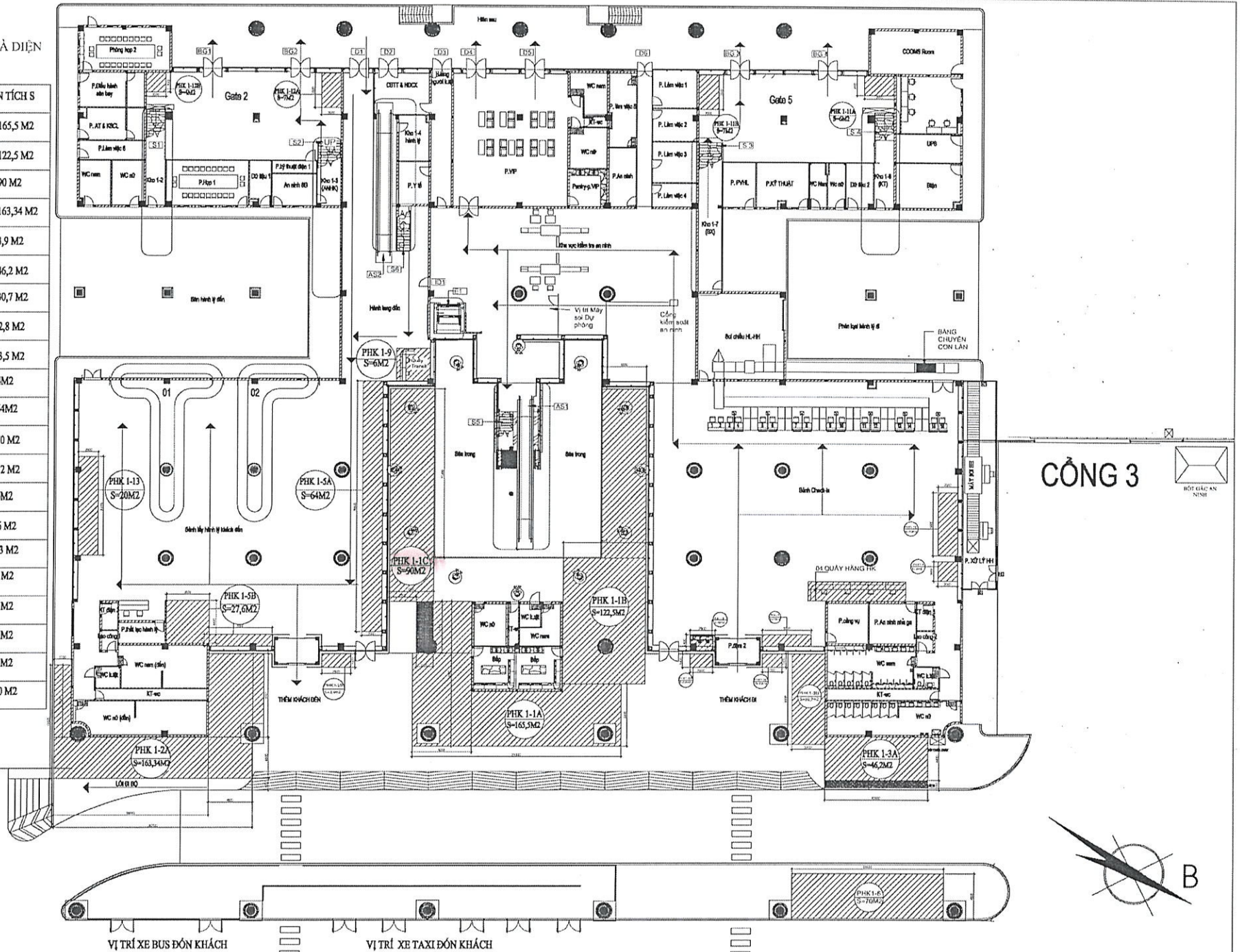
PHỤ LỤC 03A: SƠ ĐỒ MẶT BẰNG PHI HÀNG KHÔNG TẦNG 1- NHÀ GA T1 - CẢNG HÀNG KHÔNG PHÙ CÁT
